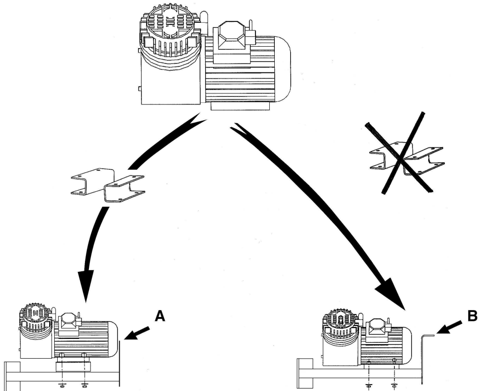
ANCIEN SUPPORT DE POMPE OLD PUMP SUPPORT ANTIGUO SOPORTE DE BOMBA EHEMALIGE PUMPESTÜTZE
